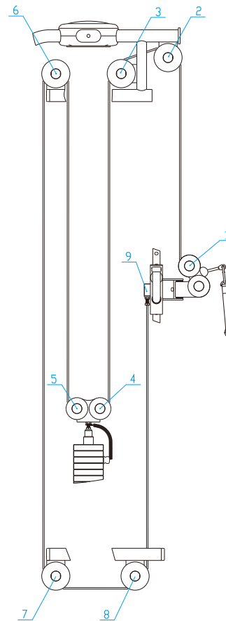
可调式滑轮训练方位钢丝绳走线图
